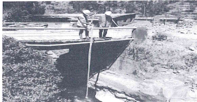
Tomando la Medición de la altura del Galibo del Puente existente
