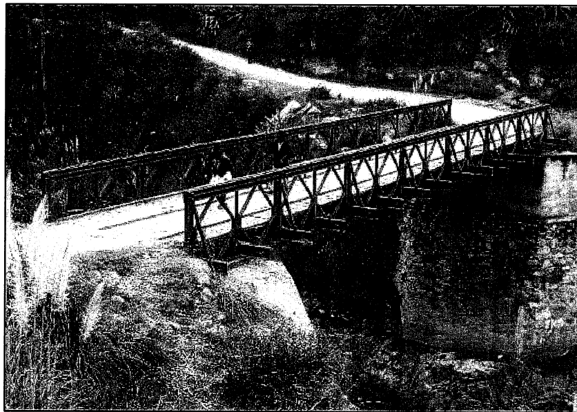
Fotog. 01: Puente San Pedro y sus estribos
