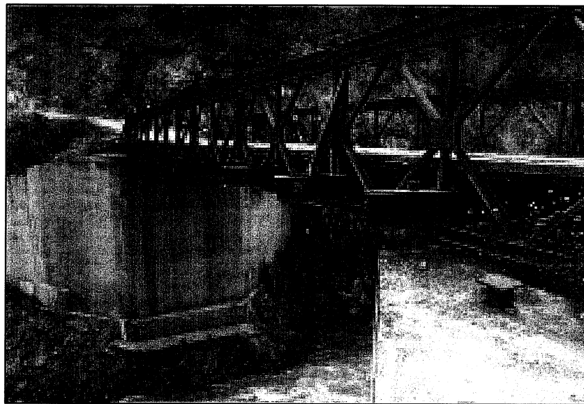
Fotog. 02: Vista del estribo izquierdo del puente
