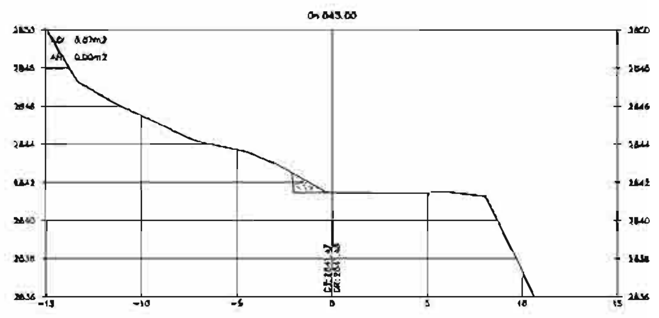
PLANO SECCION TRANSVERSAL ESC. 1:1/100
