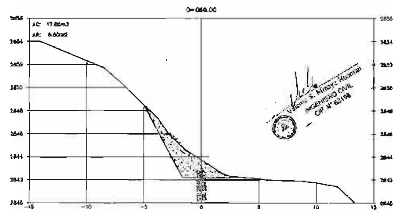
PLANO SECCION TRANSVERSAL ESC. 1:1/100
