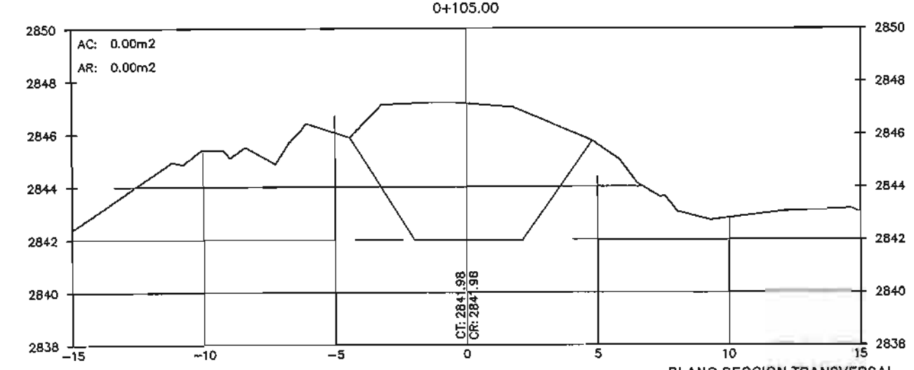
PLANO SECCION TRANSVERSAL ESC. H=1/200
