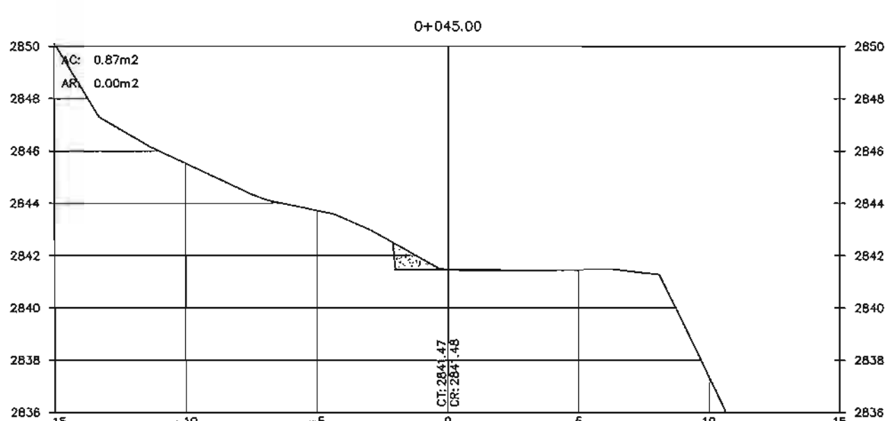
PLANO SECCION TRANSVERSAL ESC. H=1/200
