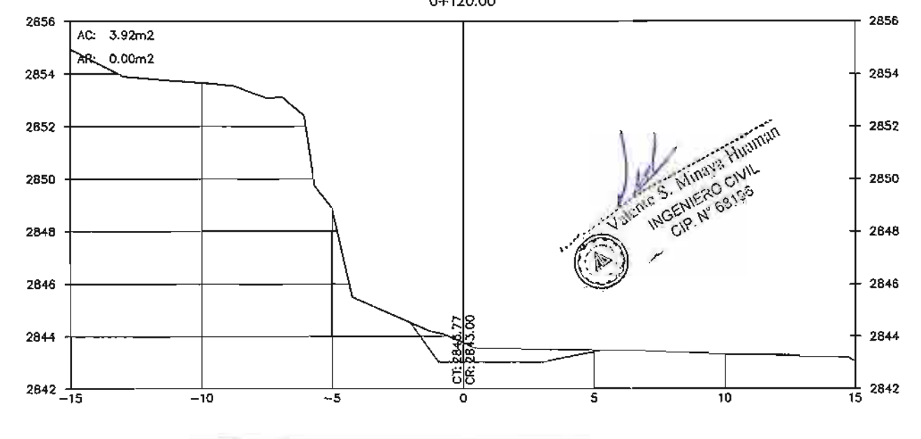
PLANO SECCION TRANSVERSAL ESC. H=1/200
