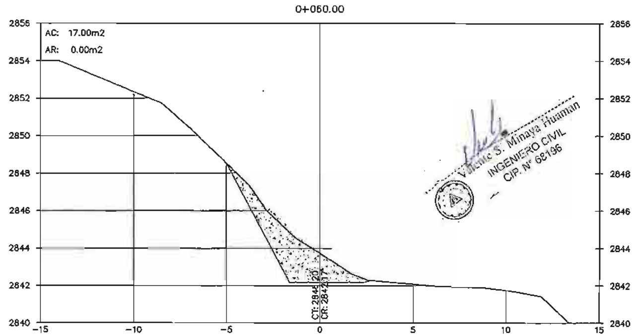
PLANO SECCION TRANSVERSAL ESC. H=1/200
